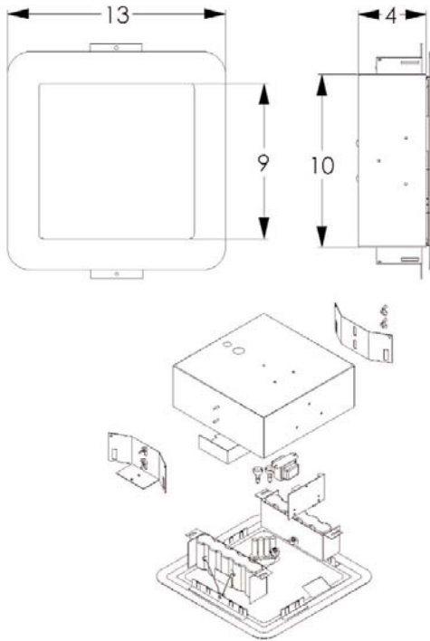
DIMENSIONS
